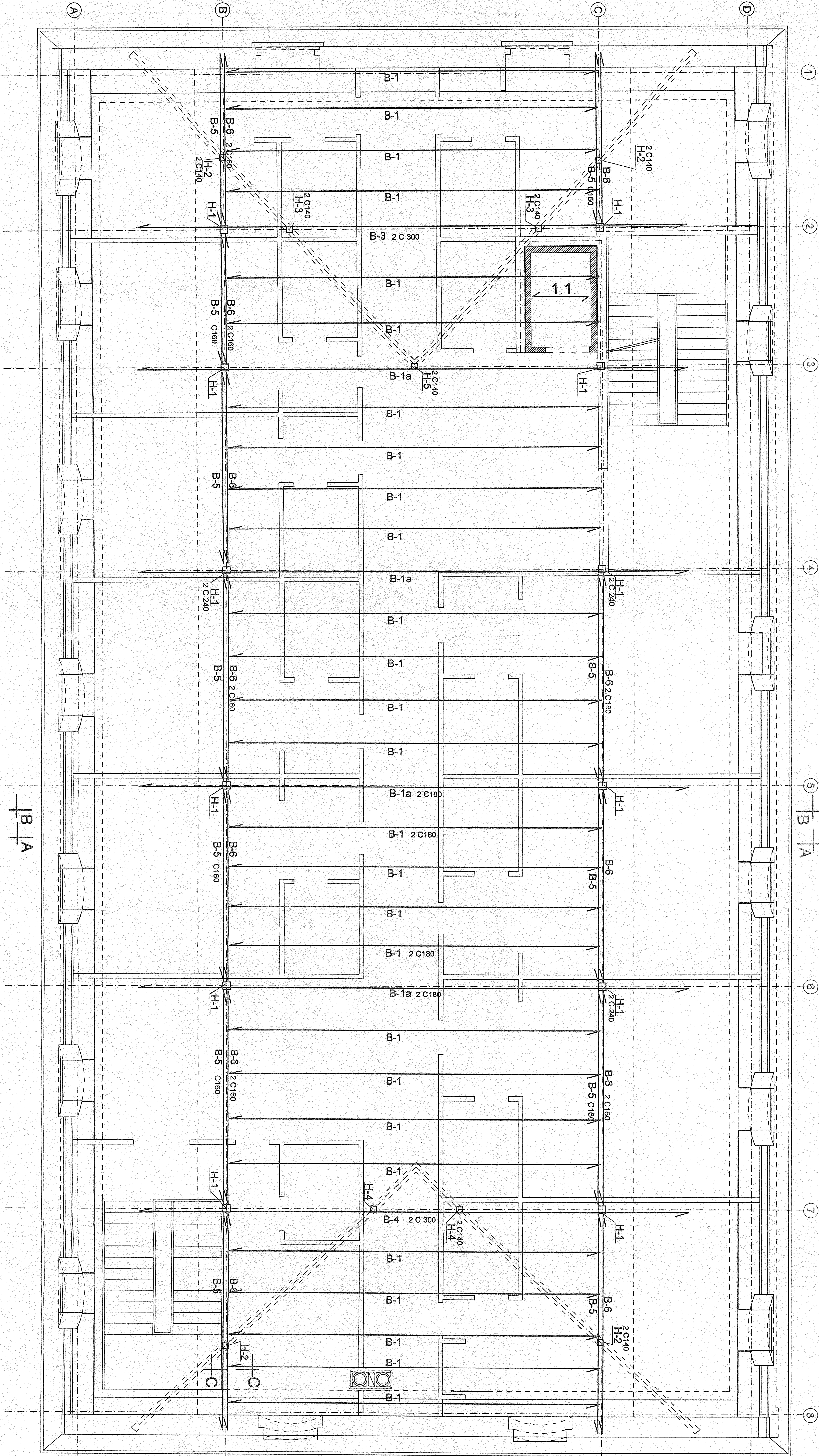
RZUT KONSTRUKCYJNY PODDASZA 1:50
